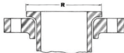
Lap-Joint
